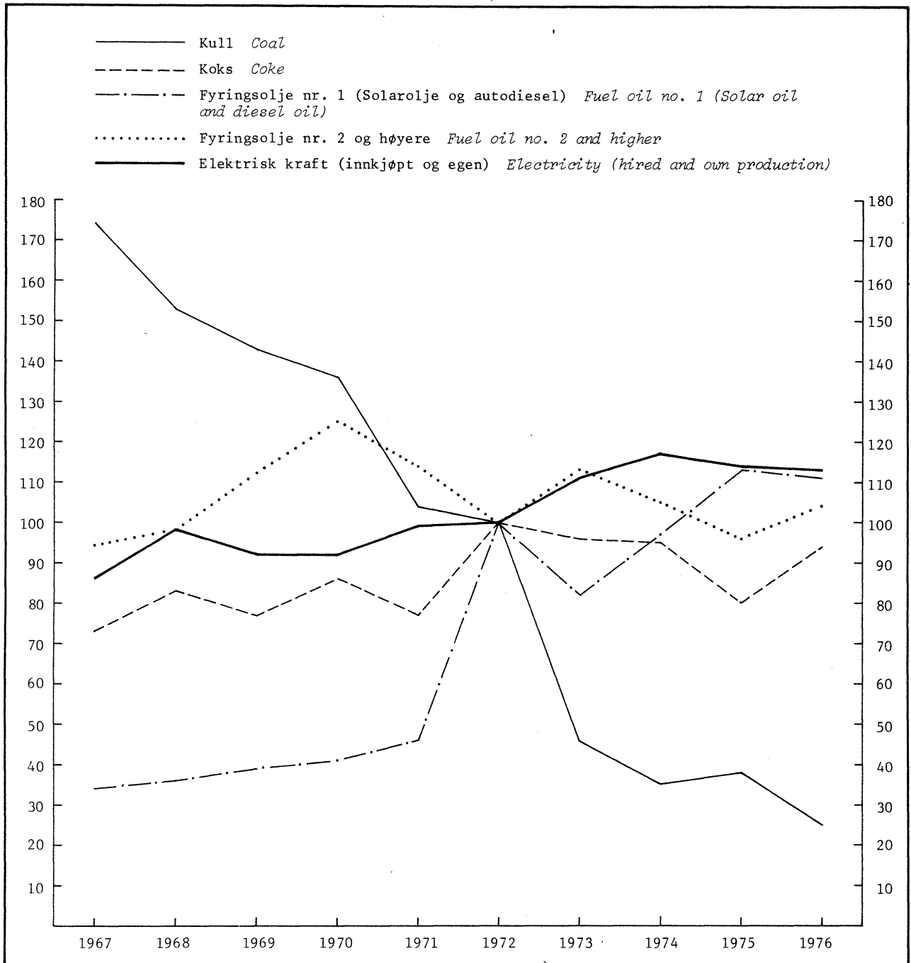
FIGUR 12. FORBRUK AV BRENSEL OG ELEKTRISK KRAFT 1967-1976. STORE BEDRIFTER. RELATIVE TALL 1972 = 100 (BEREGNET UT FRA MENGDEOPPGAVENE) CONSUMPTION OF FUEL AND ELECTRIC ENERGY 1967-1976. LARGE ESTABLISHMENTS. PROPORTIONATE FIGURES 1972 = 100 (CALCULATED ON DATA OF QUANTITY)
