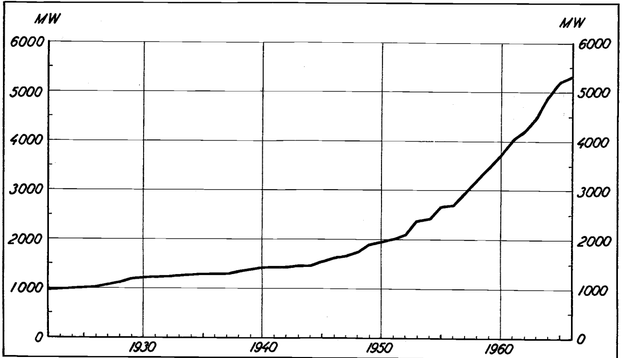
Diagram 35. Utbygd vannkraft. 1922—1966. MW. Developed water power. 1922—1966. MW.
