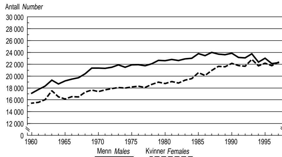
Døde menn og kvinner. 1960-1997 Deaths, males and females. 1960-1997
